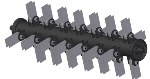
Fig. 2 Dettaglio rotore con coltelli dritti a doppio taglio Rotor with double straight knives detail Rotordetail mit geraden zweischneidigen Messern
