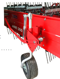
Fig. 2 Dettaglio gruppo montante con ruota e leva di registrazione dell'altezza Upright group detail with wheel and height adjusting lever
