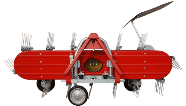
Abb. 7 NEW FALCON mit Dreieck-Anschluss mit Stange und einem Tastrad
